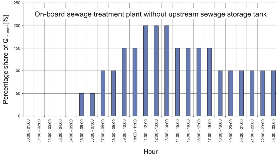
Фигура 2: Дневен график за подаване на отпадъчни води към бордова станция за пречистване без резервоар за отпадъчни води преди нея
