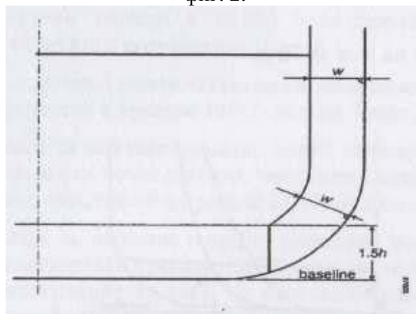
Фигура 2 - Гранични линии на товарните танкове за целите на
