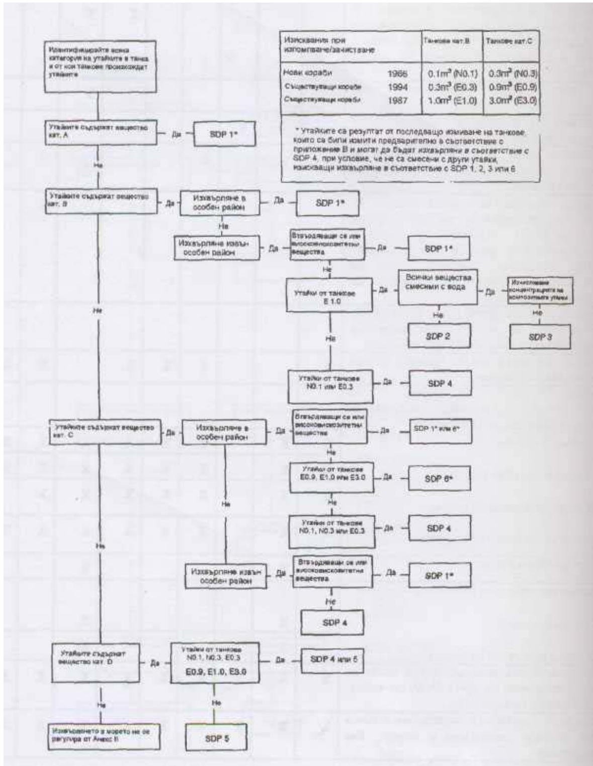
Бележка: Това е технологична схема, ясно представяща изискванията приложими за нови и съществуващи кораби. Технологичната схема за определен включва единствено частите, приложими за този кораб.
